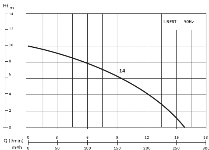
Courbes et performances de la pompe n = 2900 \text{ 1/min}
