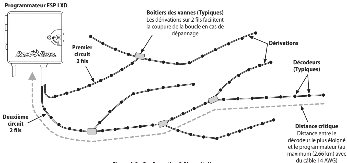
Figure A.2 - Configuration 2 fils en étoile
