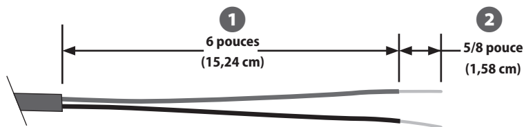
Figure H.2 - Épissure du câble 2 fils
