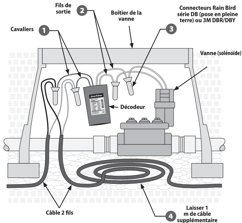
Figure H.3 - Câblage typique d'un décodeur de terrain
