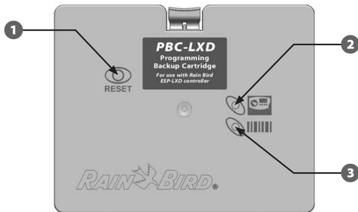
Figure E.1 - Cartouche de sauvegarde des programmes (PBC-LXD)
