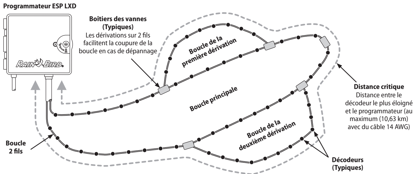
Figure A.3 - Décodeurs et vannes en configuration 2 fils en boucle
