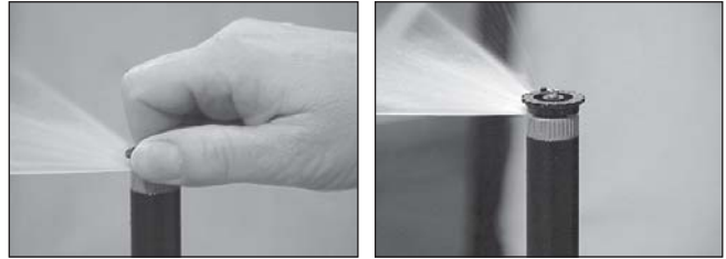
Réglage du secteur d'arrosage très accessible. opération facile à sec ou en fonctionnement.
