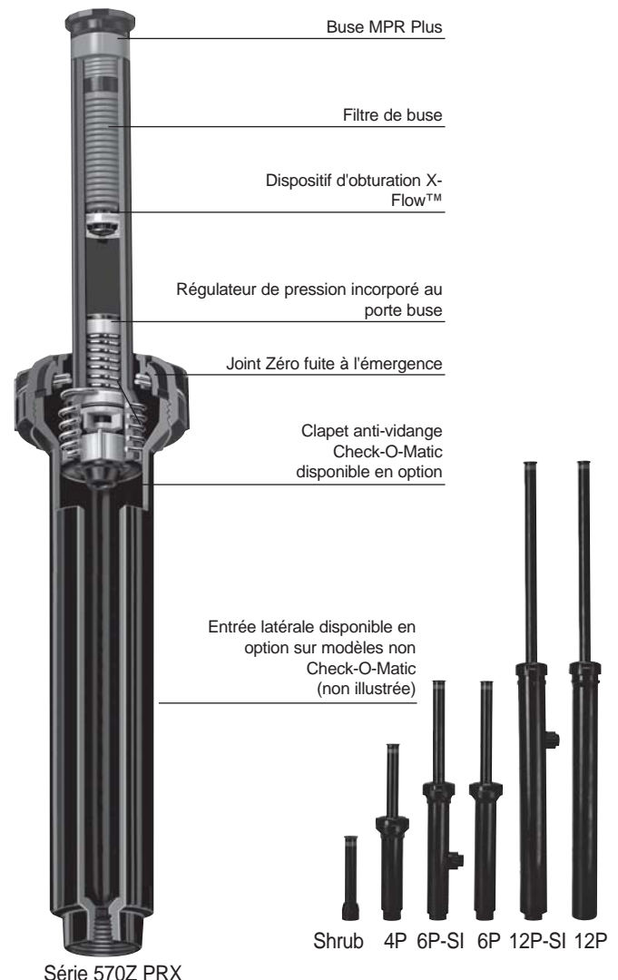
Série 570Z PRX
