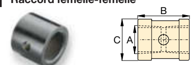
19 Raccord femelle-femelle
