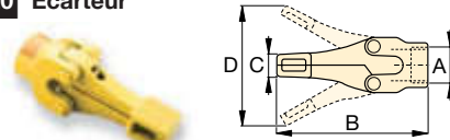
20 Ecarteur
