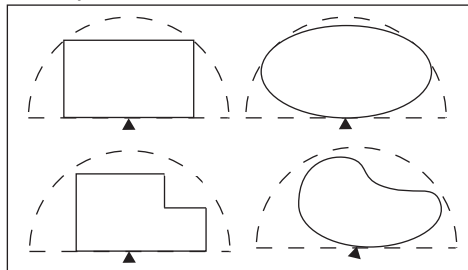
▲ centrale de détection Aqualarm --- rayon d'action de 7m d'Aqualarm
