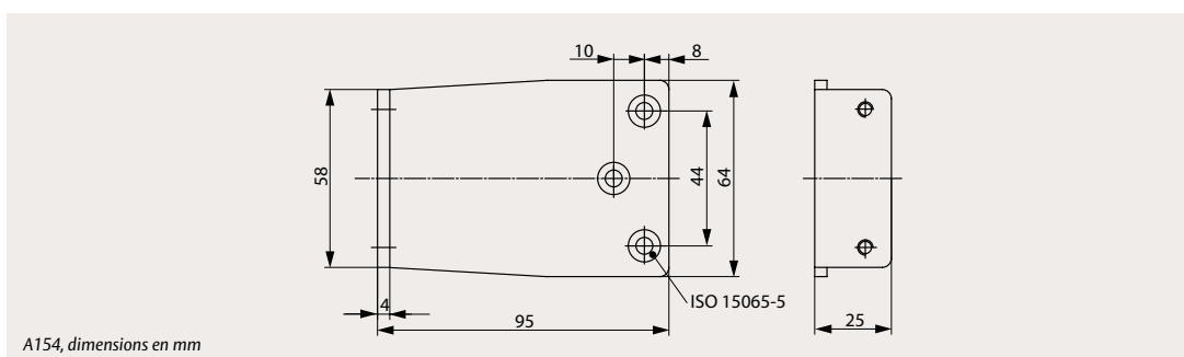
DC110, dimensions en mm
