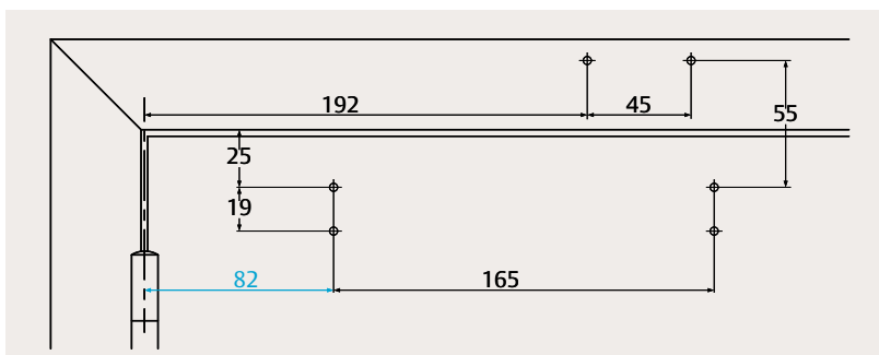
Bras compas, EN 3 dimensions de fixation
