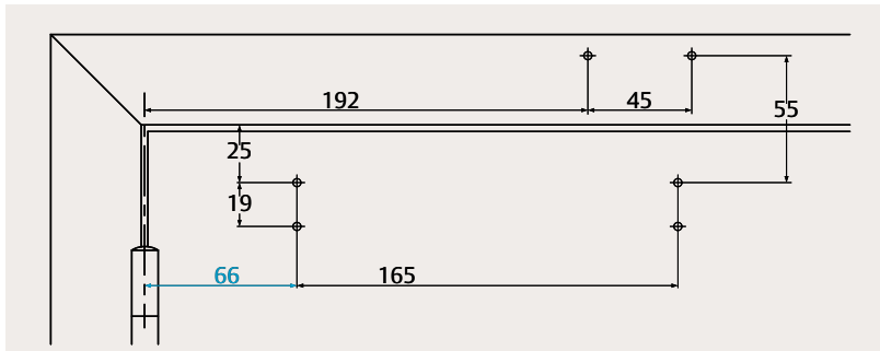
Bras compas, EN 2 dimensions de fixation
