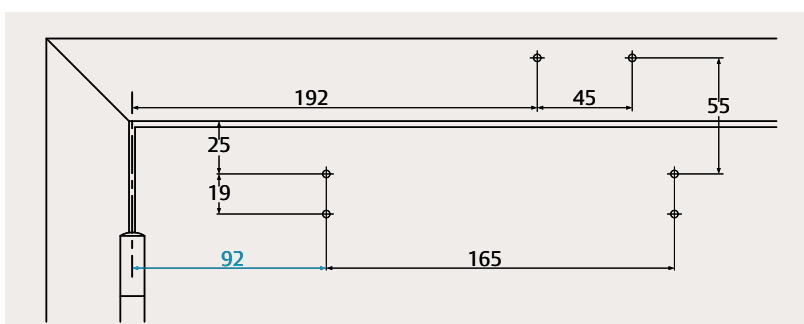
Bras compas, EN 4 dimensions de fixation
