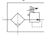
Symbole Filtre-régulateur
