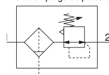
Filtre-régulateur avec fonction purge de pression
