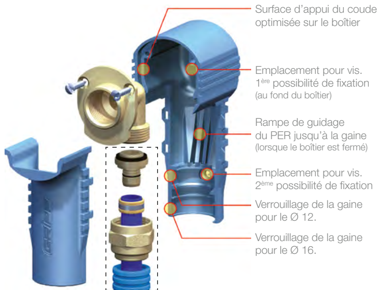
Raccordement au tube PER. Raccord à prévoir selon DN.
