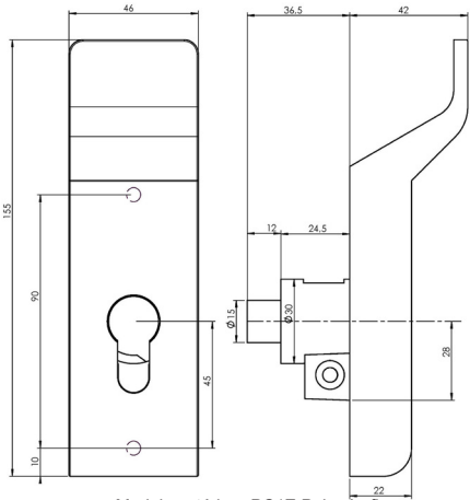
Module extérieur PC1E Poignée fixe
