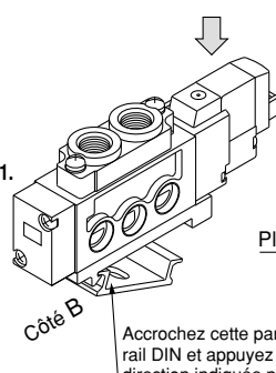
Fig. 1 Procédure de montage de l'embase
