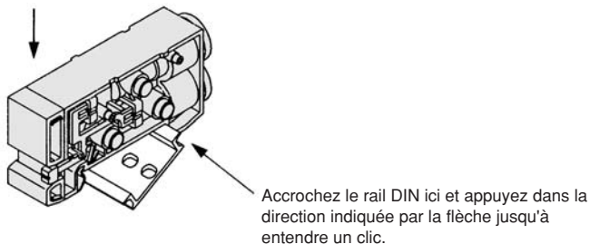
Fig. (1) Procédure de montage du bloc
