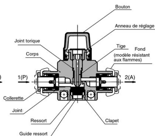
Valve 3/2/Série VHK3
