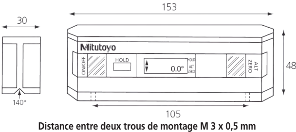
Distance entre deux trous de montage M 3 x 0,5 mm
