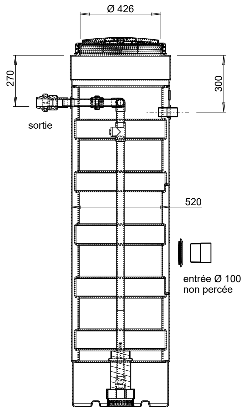
COUPE A-A
