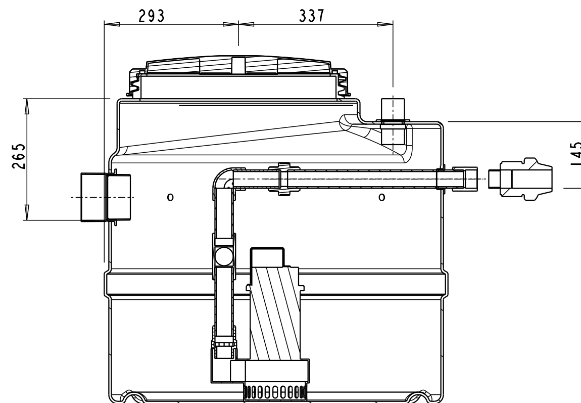
COUPE A-A
