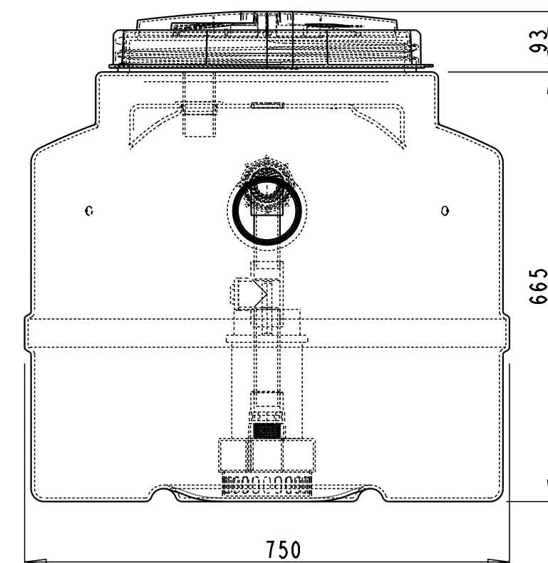
COUPE D-D
