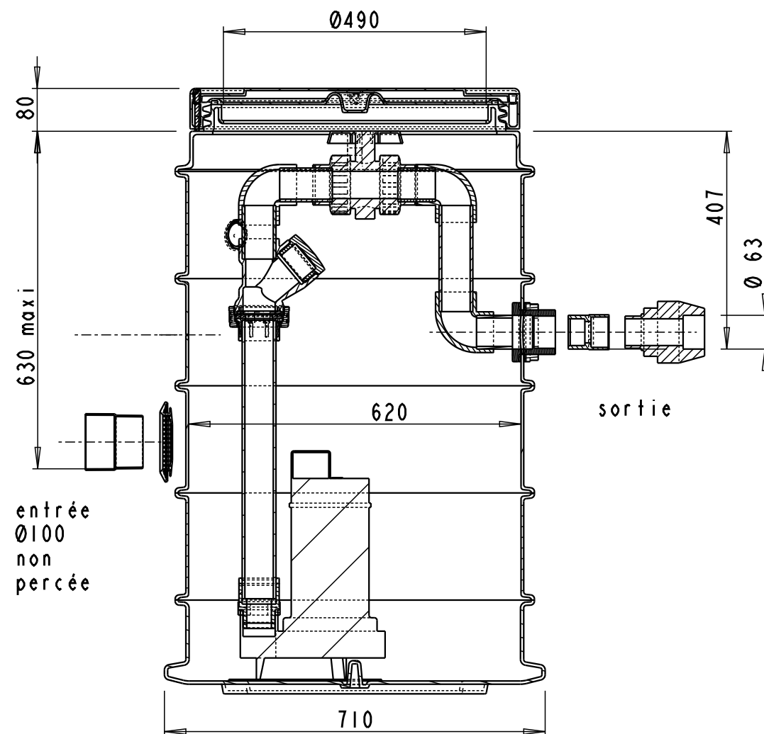
COUPE D-D
