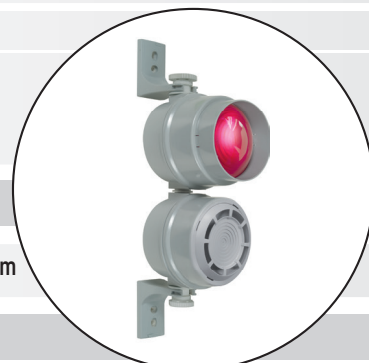
Feu fixe à LEDs 890 associé à une sirène puissante (réf. 190, voir page 216)
