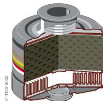
Filtre Dräger Rd40 Vue en coupe
