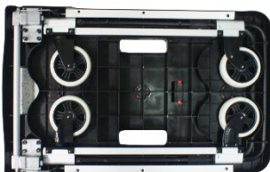
Ruedas plegables
