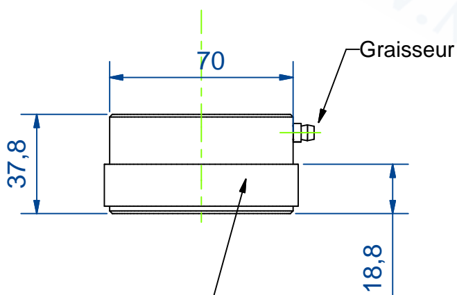
Roulement à rouleaux coniques en partie interieure ref:30305
