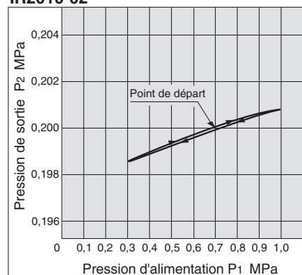
IR2020-02
