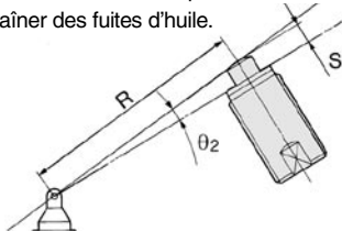
Conditions d'installation de la masse pivot libre (mm)
