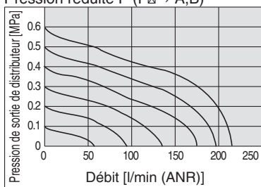
Pression réduite A1 (P 0 → A), Pression réduite B1 (P 0 → B)
