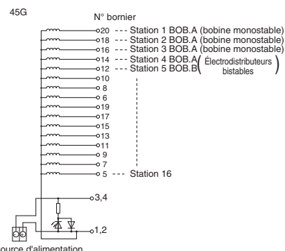
Câble plat 10GD/16GD (câblage PC)
