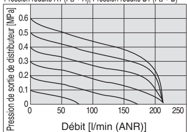
SV3000 Pression réduite P (P 0 → A,B)
