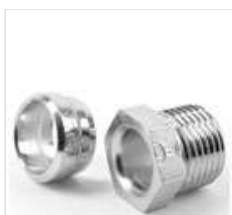
Composants de raccords DIN Ermeto pour les raccords de tubes hydrauliques haute pression
