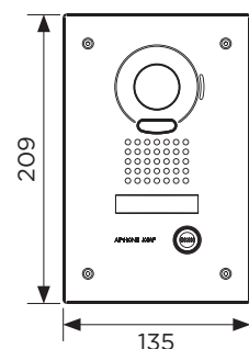
JODVF Encastrement : 180 x 110 x 45
