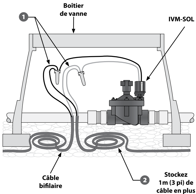
Câblage IVM-SOL-vanne typique
