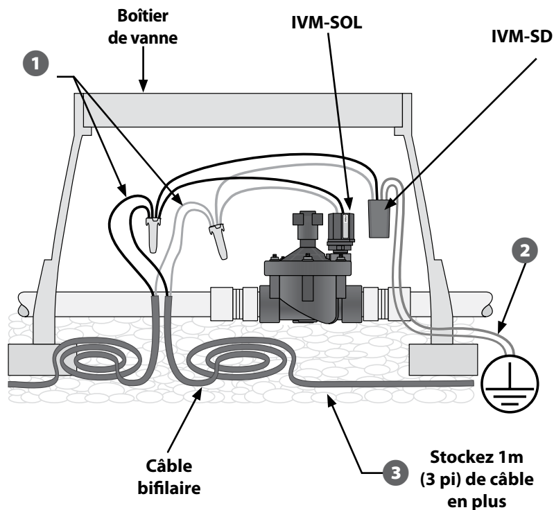
Câblage IVM-SD typique
