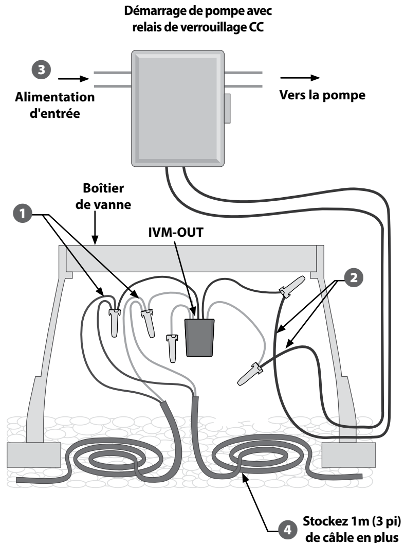
Câblage IVM-OUT-relais de démarrage de pompe typique
