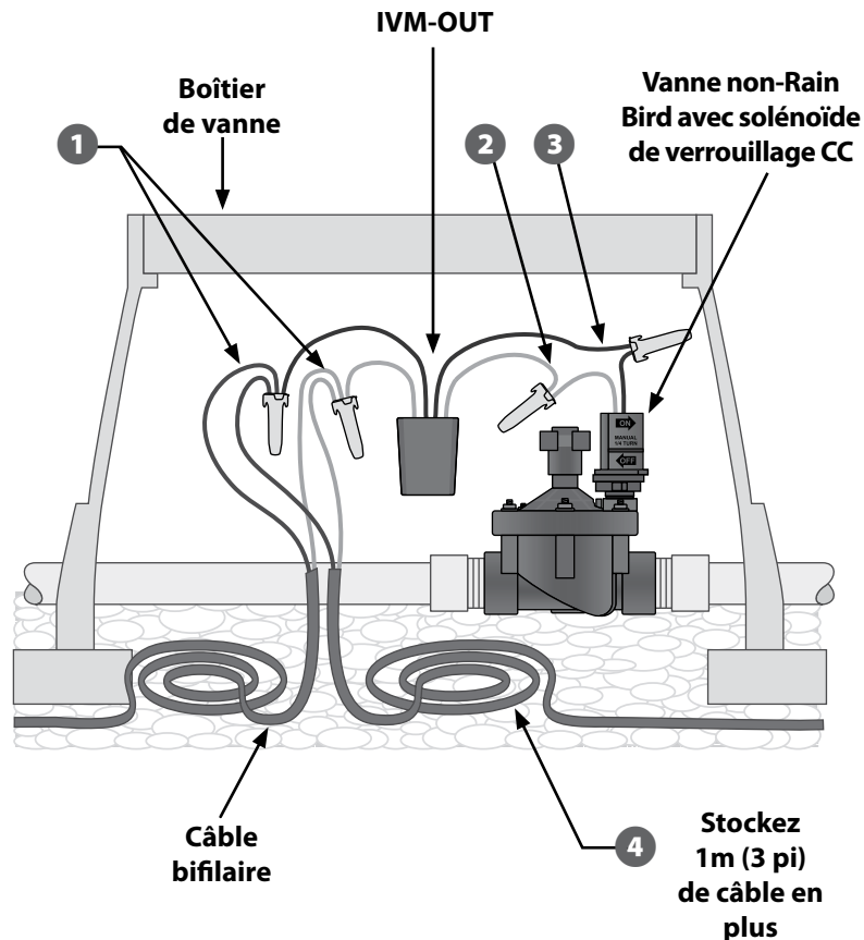
Câblage IVM-OUT typique
