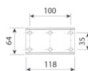
Support fixation moteur
