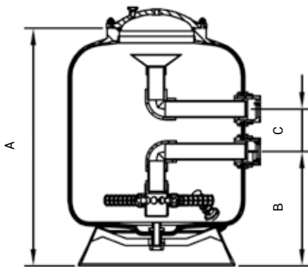
Raccord fileté Ø 500 - Ø 600 - Ø 750 - Ø 900 - Ø 1050-2"
