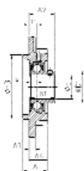
USFC200
