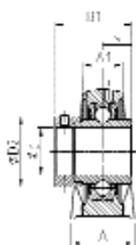
EXPLE200
