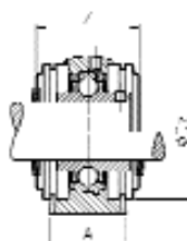
UCPLE200CO(CC)
