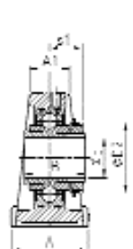
UKPAE200H
