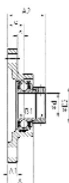
ESFLE200
