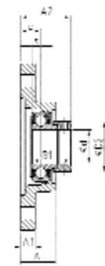
ESFL200
