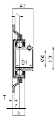
USPFE200
