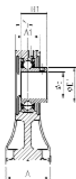
USPH200
