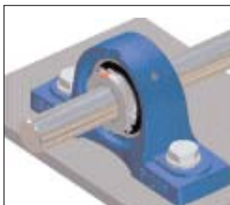
5. Bloquer le manchon de serrage (plier une languette de la rondelle-frein dans une rainure de l'écrou à encoches).
