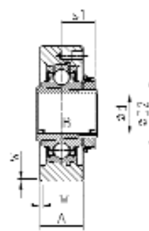
UKC200H UKC300H
