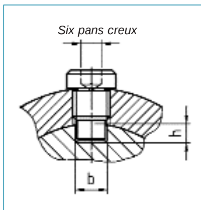
Dimensions de la rainure d'arbre
