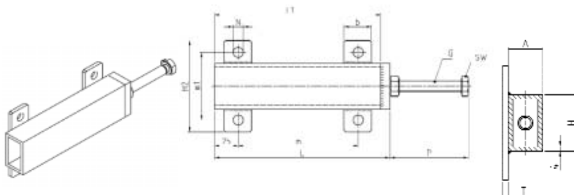
SPR11+21
