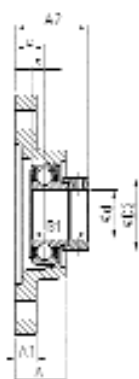
ESFL200
