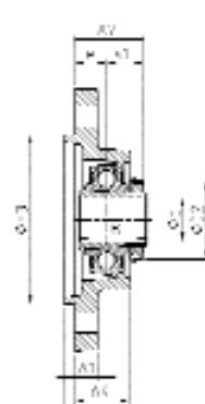
UKFLZ200H
