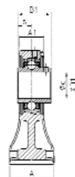
UCPH200
