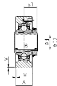
UKC200H UKC300H
