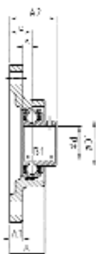
USFLE200
