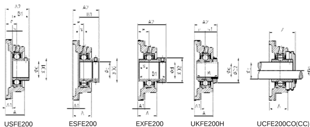
USFE200
