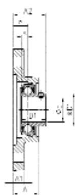
USFL200
