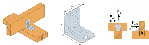
Fixation bois/bois
