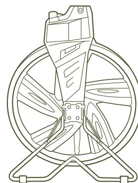
Béquille : acier et plastique Diamètre de la roue : 319,6 mm
