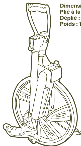
Compteur rotatif à 5 chiffres mesurant de 0 à 9 999,9 m
