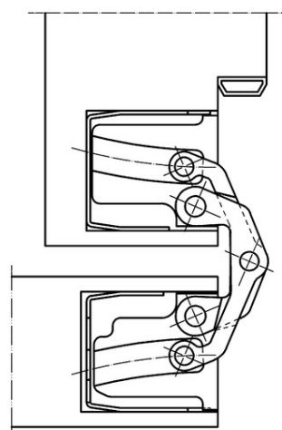
bloc-porte 180°
