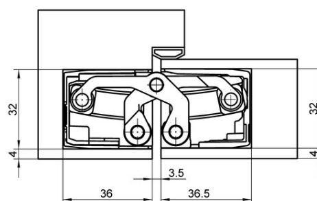
bloc-porte
