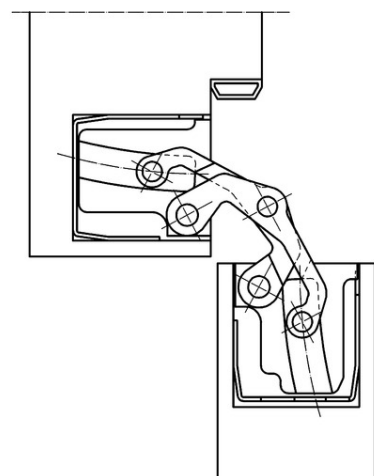
bloc-porte 90°
