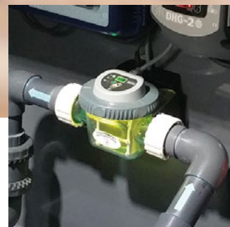
Exemple d'installation Installation of the chlorinator
